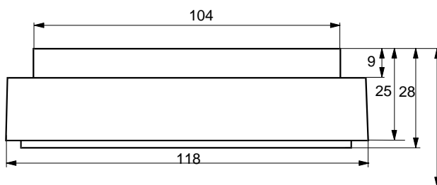
Рис. 2. Чертеж основания USB501-6 с размерами
