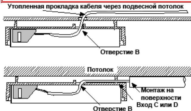
Рис. 4. Способы ввода кабеля
