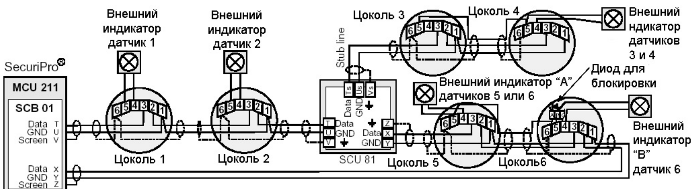
Рис. 3 Примеры подключения
