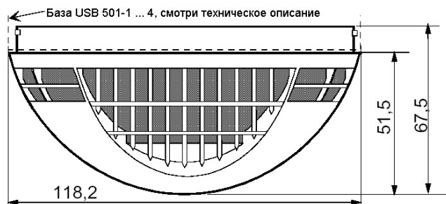
Рис. 2 Габаритные размеры
