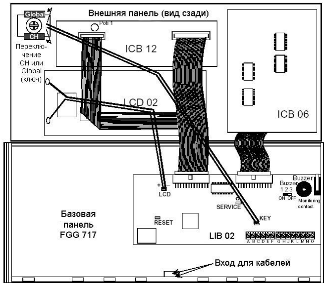
Рис. 3 Подключение MIC 734 и FGG 717
