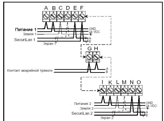
Рис. 4 MIC 734 подключение
